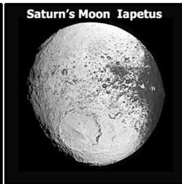
Iapetus
