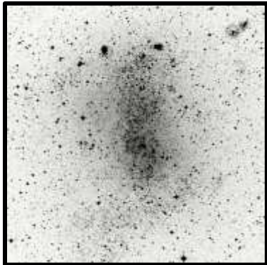
NGC6822 15'
