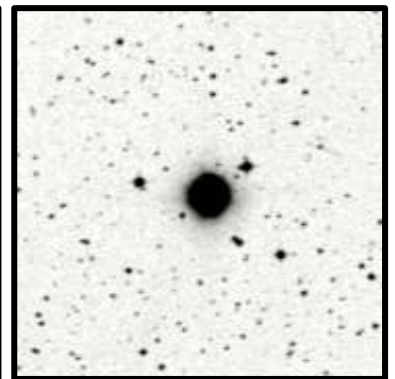
NGC6818 5'
