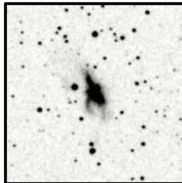
NGC6240 5'
