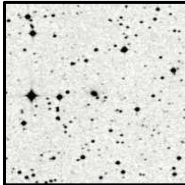
SC 7 (NGC6822) 5'
