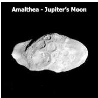
Amalthea
