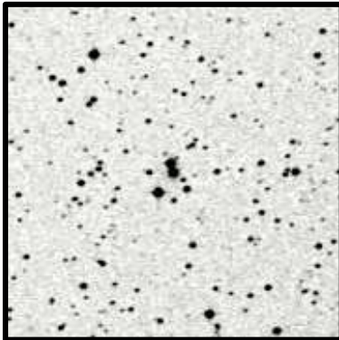
Sc 6 (NGC6822) 5'
